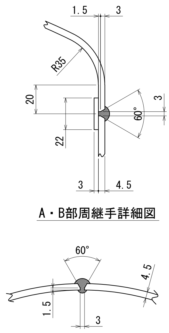
長手継手溶接部詳細図
