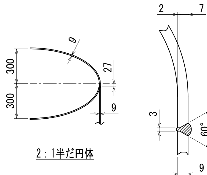
A, B部詳細図
