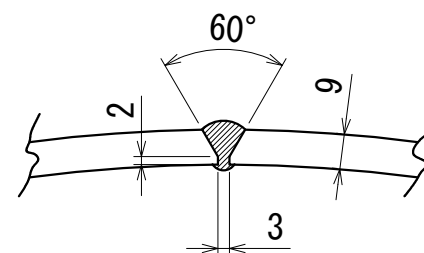
長手継手溶接部詳細図
