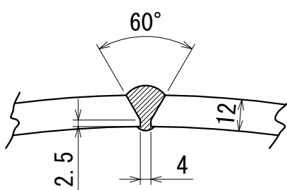
長手継手溶接部詳細図
