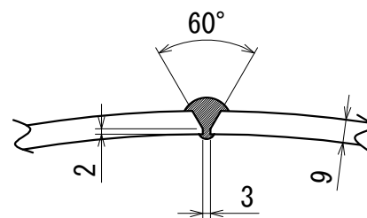
長手継手溶接部詳細図
