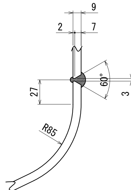
B部詳細図
