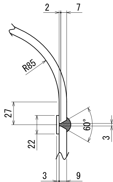
A部詳細図
