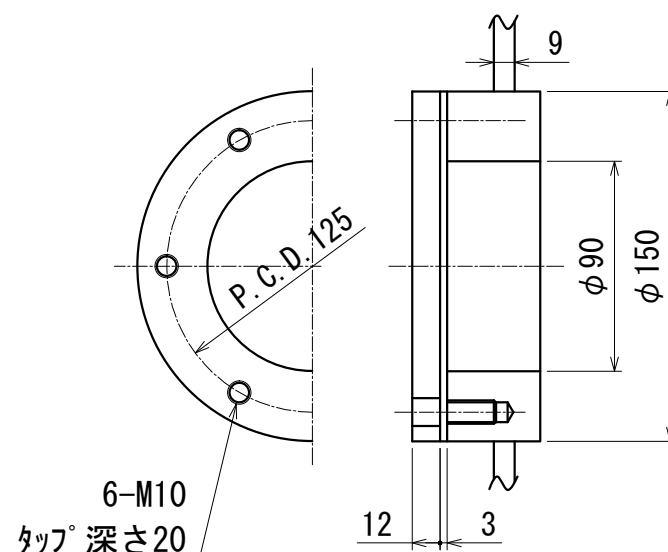
掃除口詳細図
