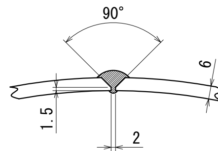
長手継手溶接部詳細図
