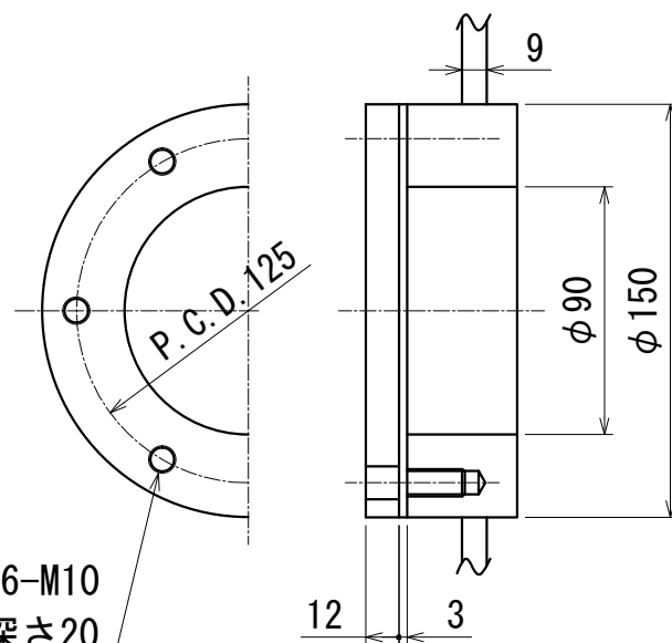
掃除口詳細図
