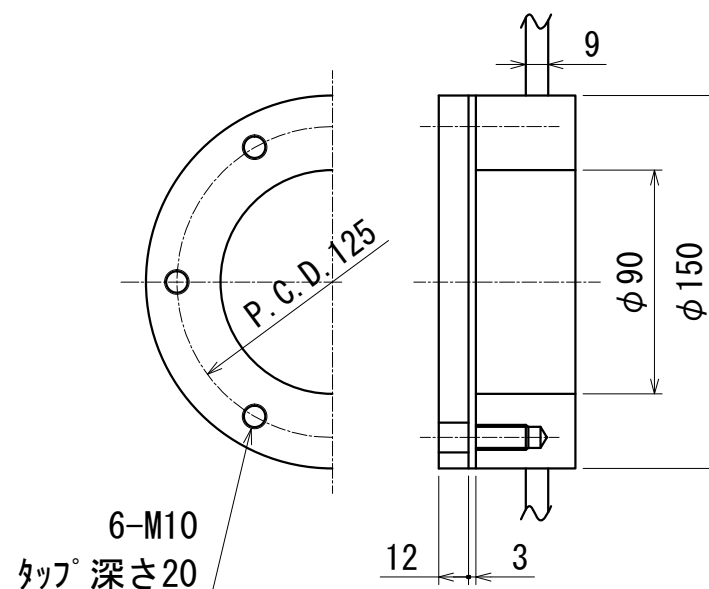
掃除口詳細図
