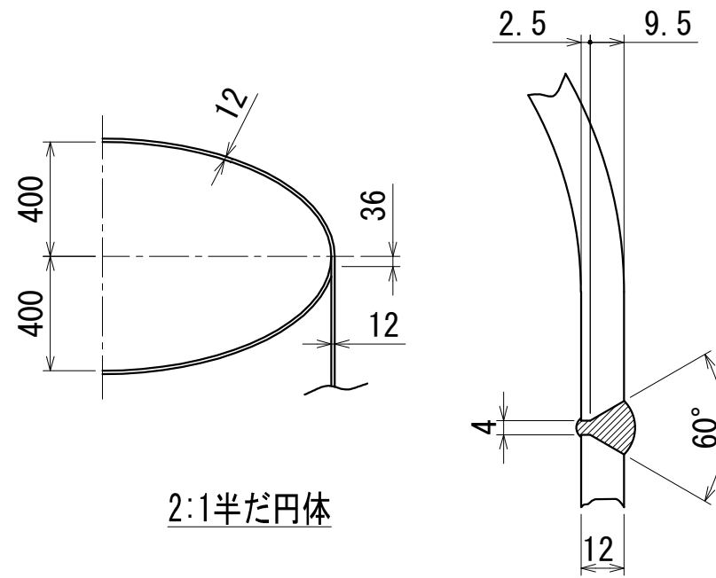
A, B部詳細図
