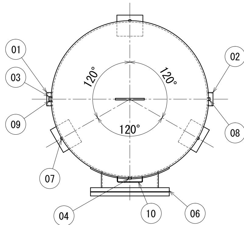
D1-D2矢視図
