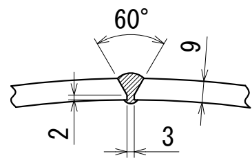
長手継手溶接部詳細
