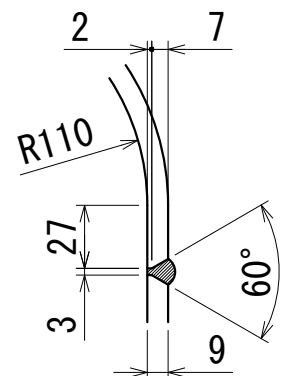
A、B部詳細
