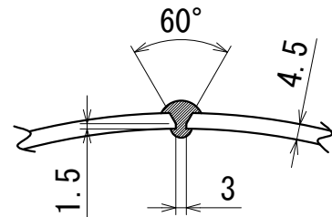
長手継手溶接部詳細図
