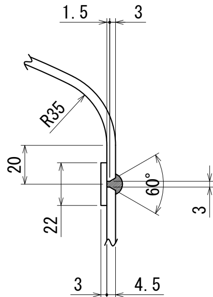
A・B部周継手詳細図
