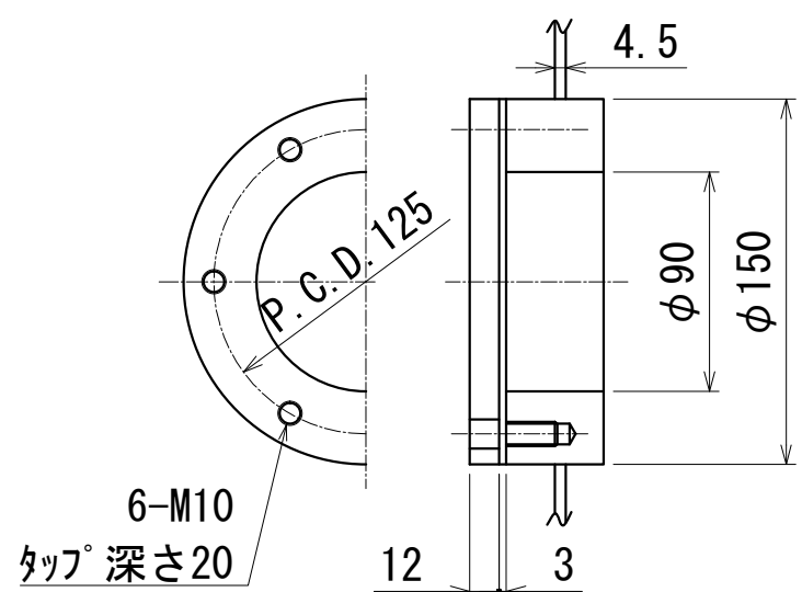
掃除口詳細図
