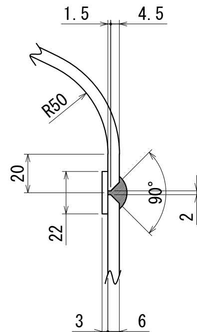
A・B部詳細図
