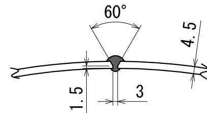
長手継手溶接部詳細図
