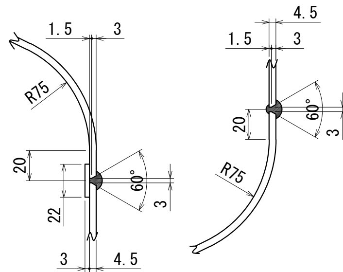
B部詳細図
