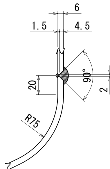
B部詳細図
