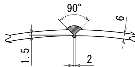
長手継手溶接部詳細図
